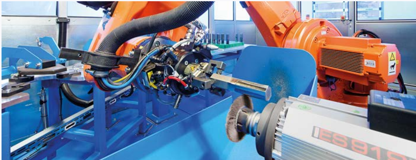
Robot di prova a Burgwald/Germania
