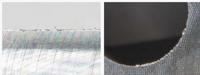
Prima della lavorazione - Bave ben definite sul bordo. Scanalature di fresatura sulla superficie.
