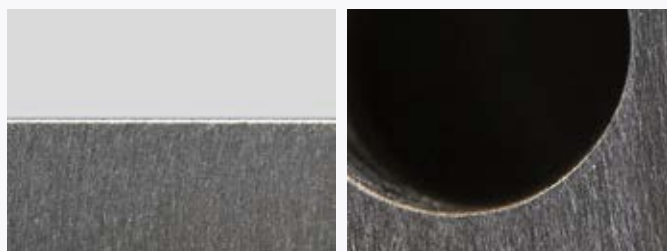
Dopo la lavorazione - Le bave sono state rimosse in modo affidabile e i bordi sono stati arrotondati. La superficie ha un aspetto uniforme e spazzolato.
